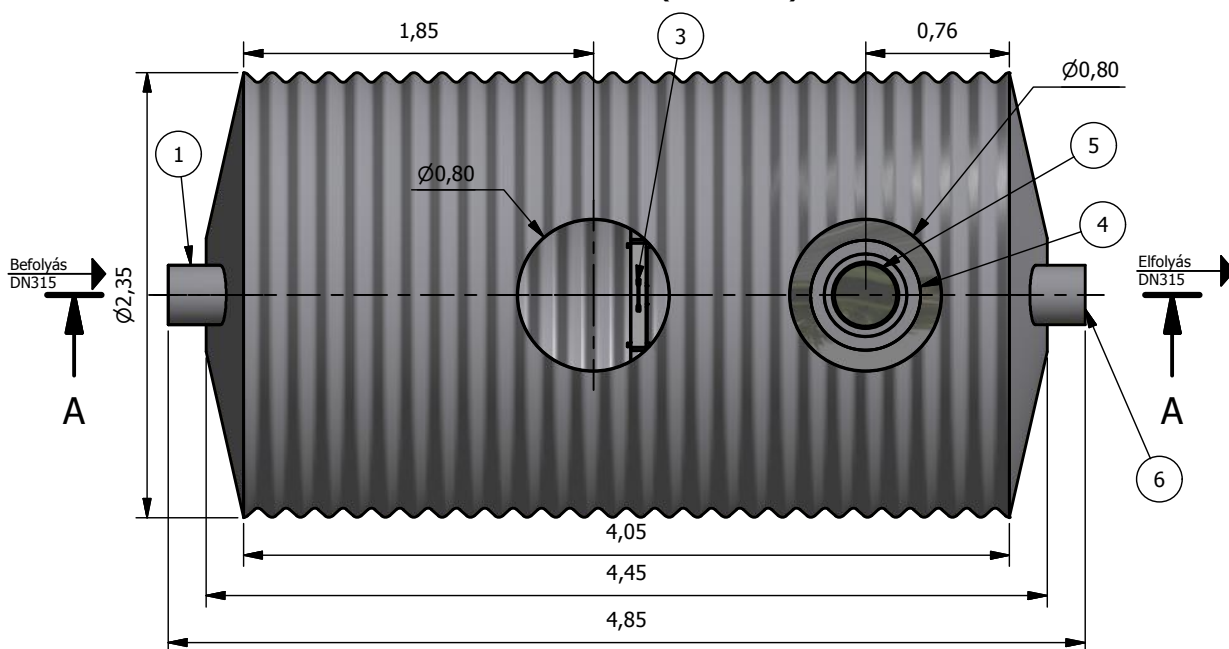
Felülnézet ( 1 : 40 )
