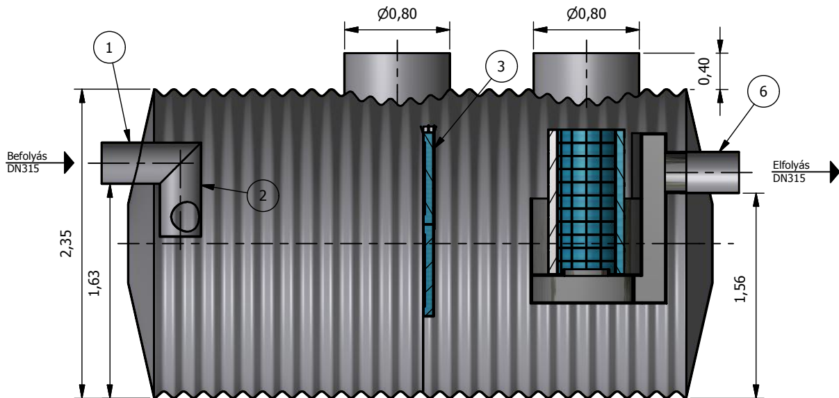
A-A ( 1 : 40 )
