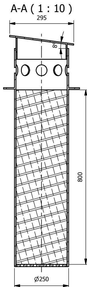
VENTUS Pipe 250 ( 1 : 10 )
