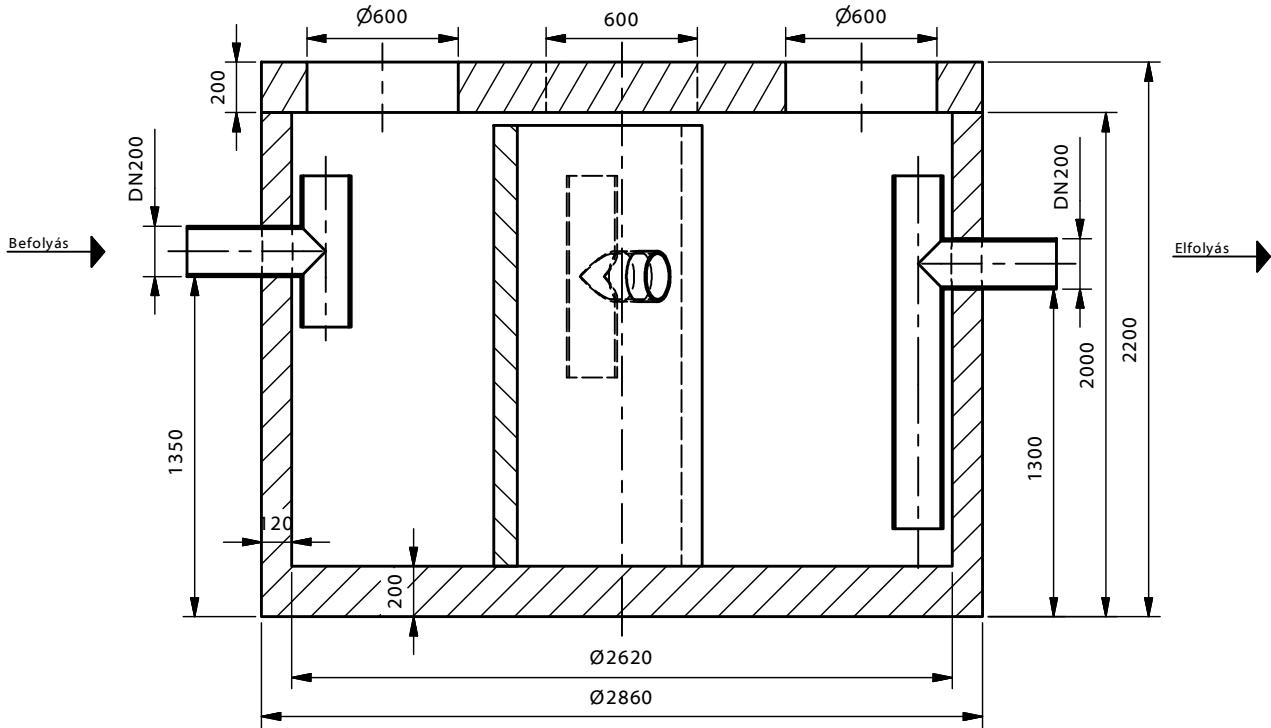
A-A ( 1 : 30 )
