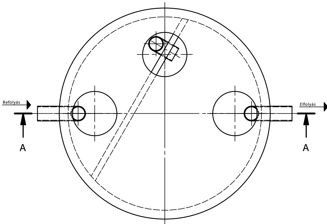
Felülnézet ( 1 : 30 )
