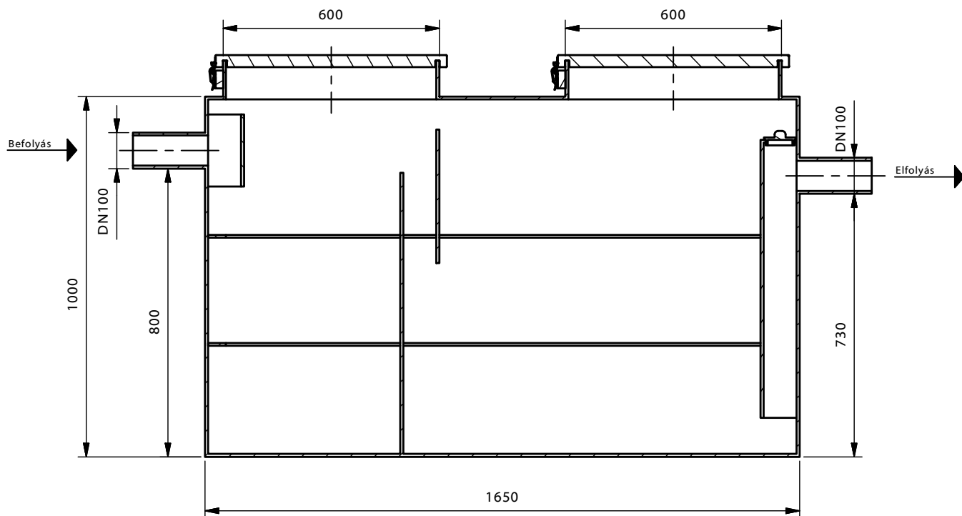
A-A ( 1 : 15 )
