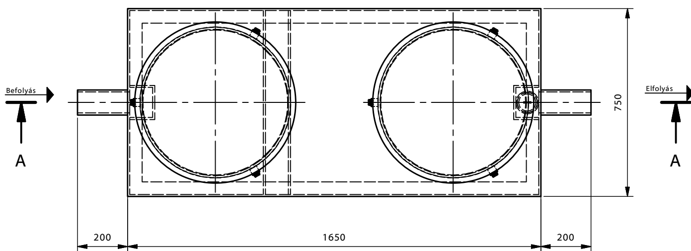
PARCO 3-P ( 1 : 50 )
