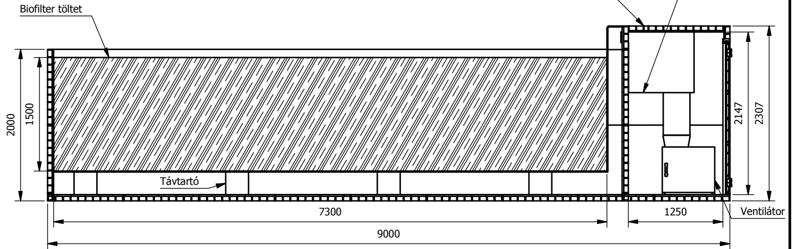
A-A ( 1 : 50 )
