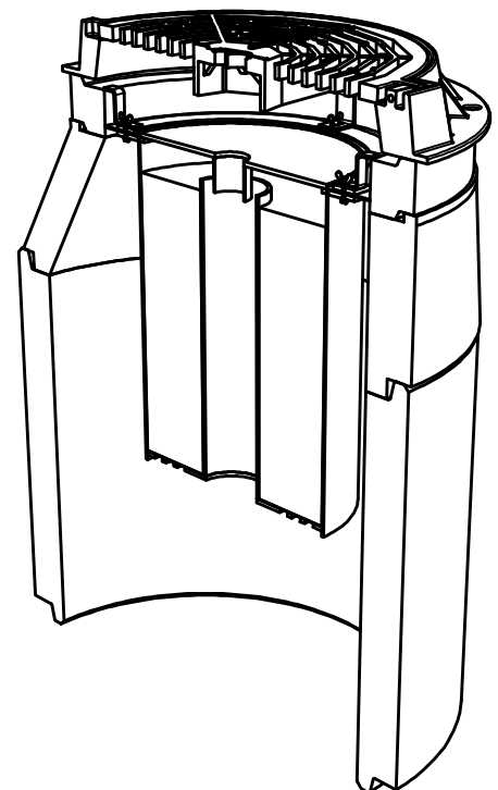
VENTUS G-10 fedlap alá szerelve ( 1 : 15 )
