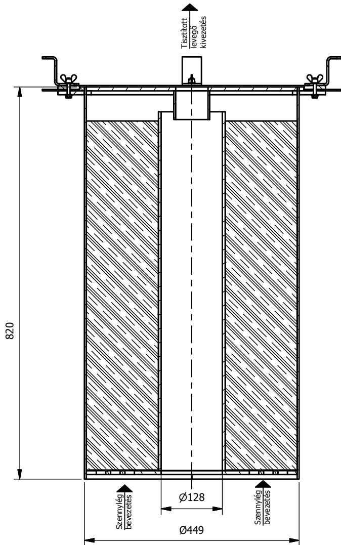
A-A (1 : 8)
