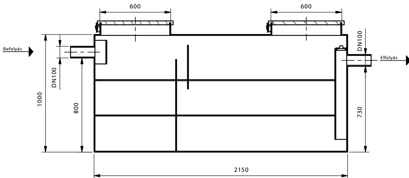
A-A ( 1 : 20 )
